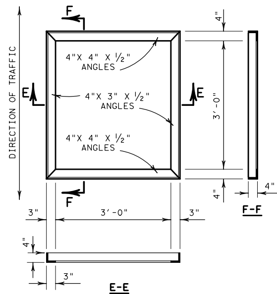
FRAME DETAIL N. T. S.
