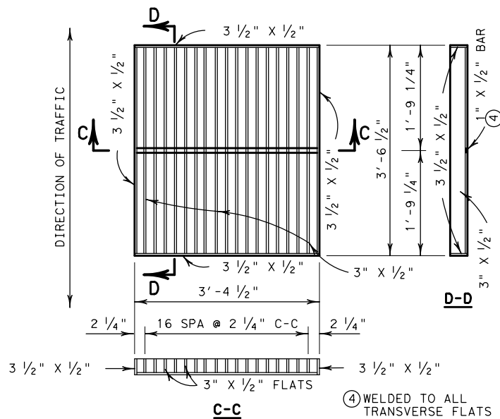
GRATE DETAIL N. T. S.
