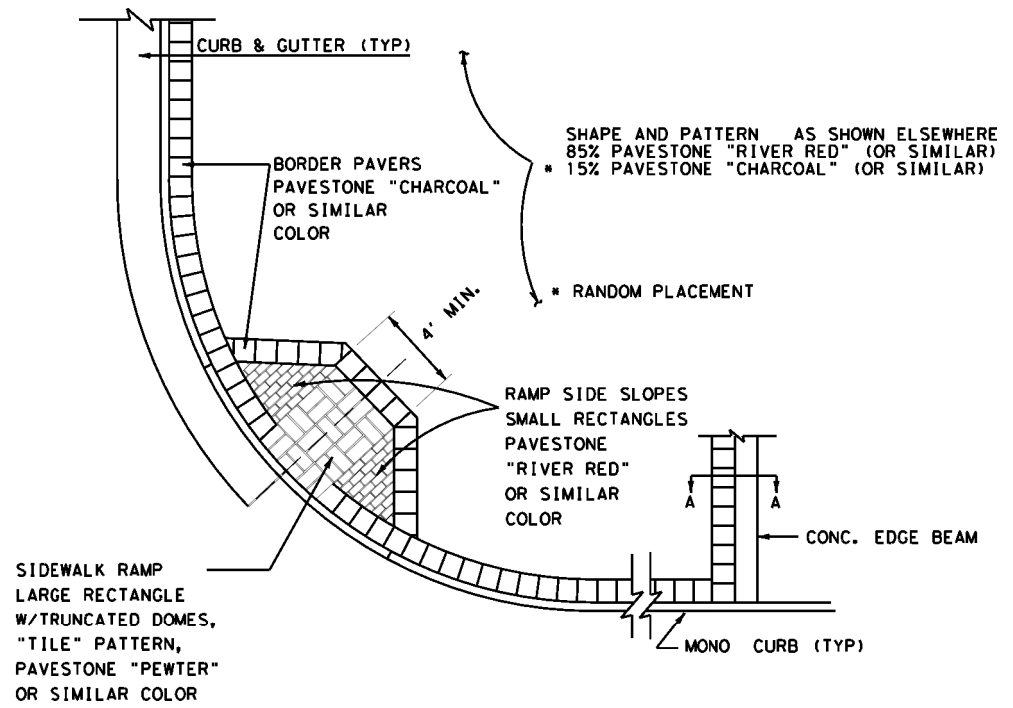
TYPICAL PAVER LAYOUT N. T. S.
