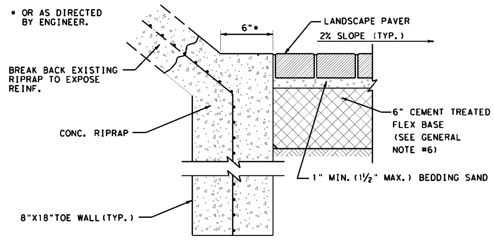
PAVER DETAIL AT RIPRAP SLOPE N. T. S.
