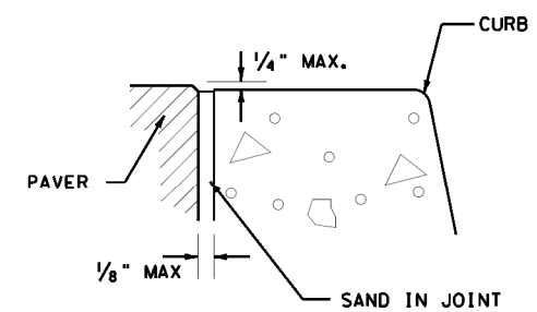
PAVER DETAIL AT CURB N. T. S.
