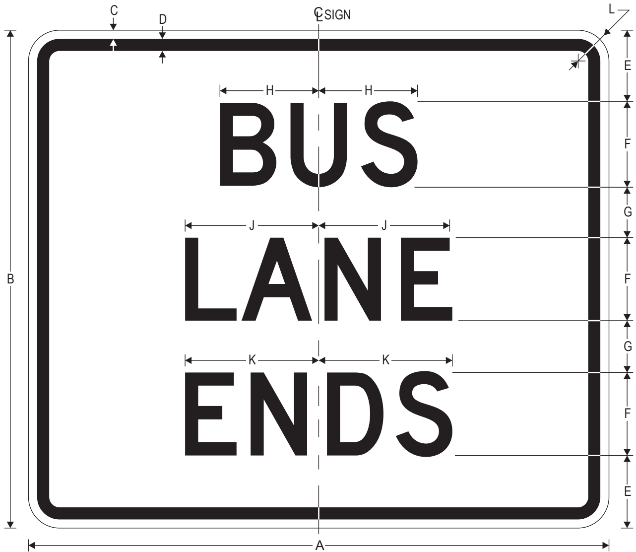
R3-15e (Overhead) BUS LANE ENDS
