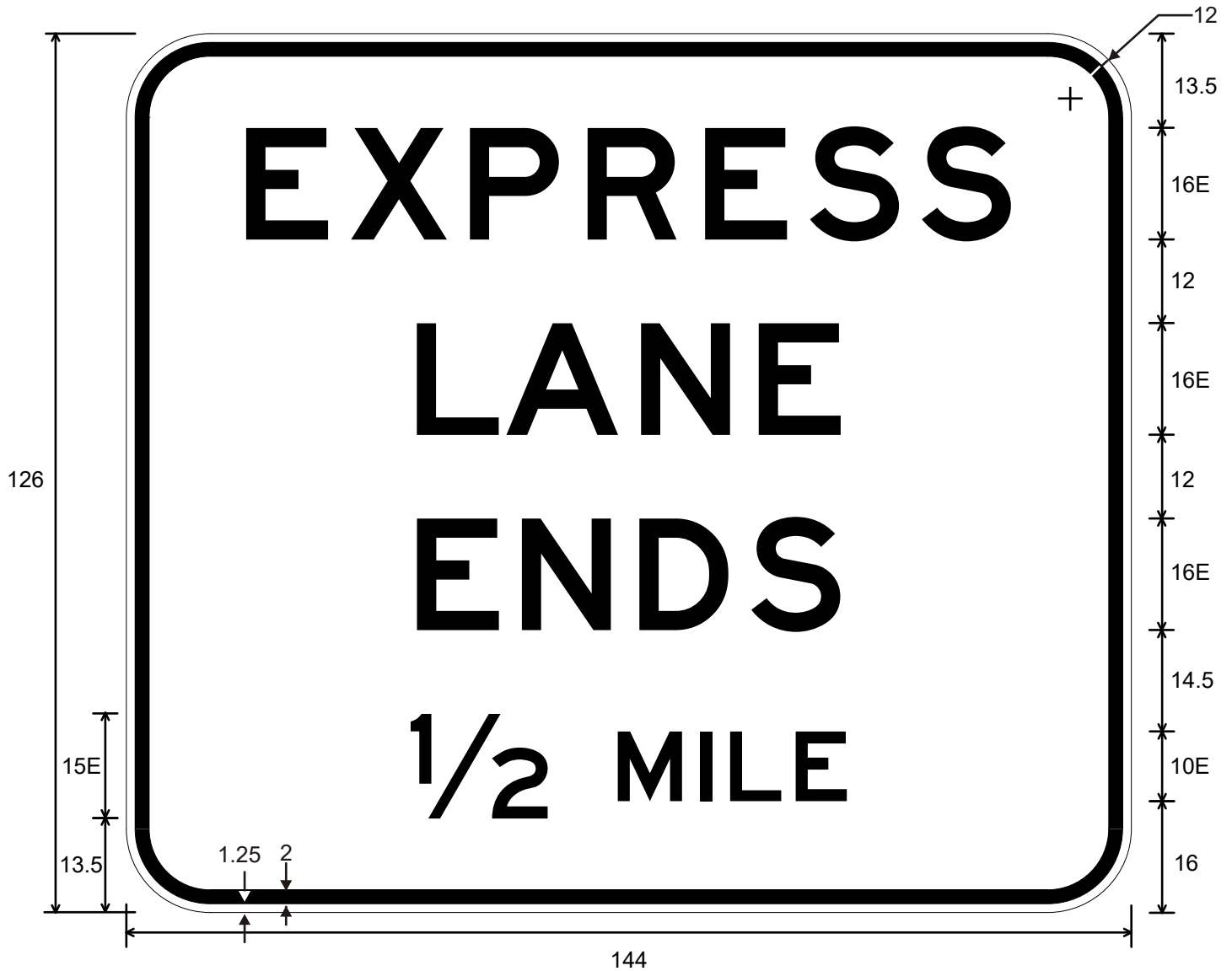
R3-42aT (Overhead) EXPRESS LANE ENDS X MILE
