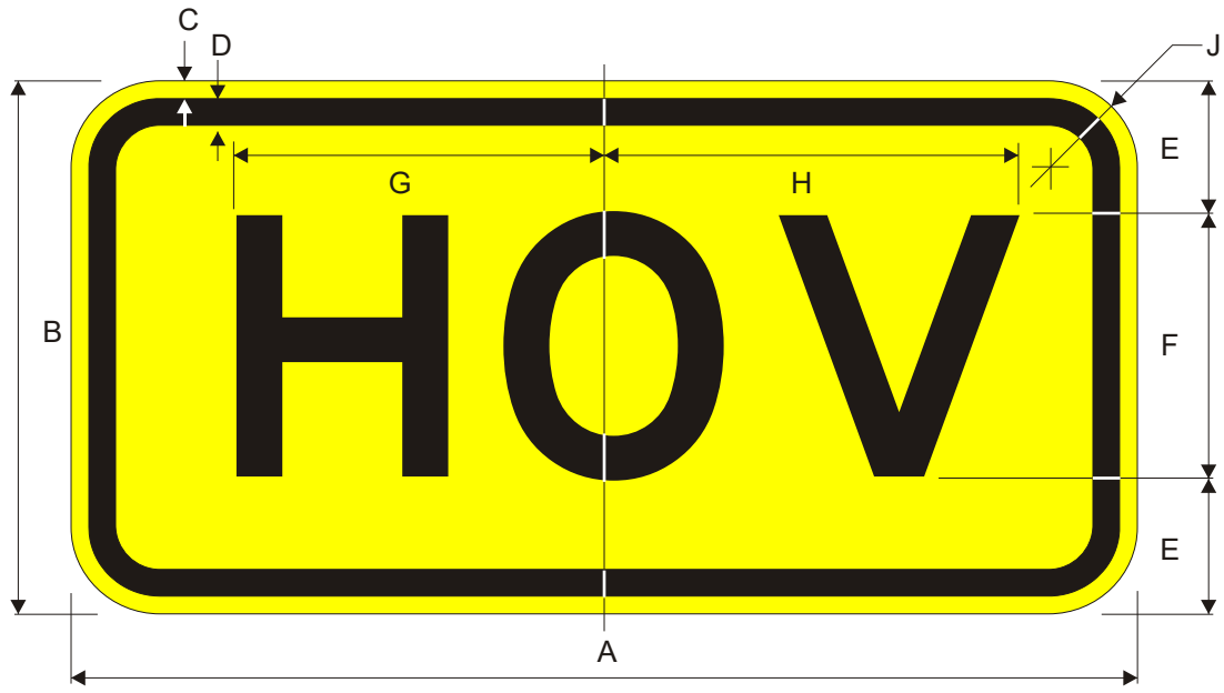
W16-11P HOV (Plaque)
